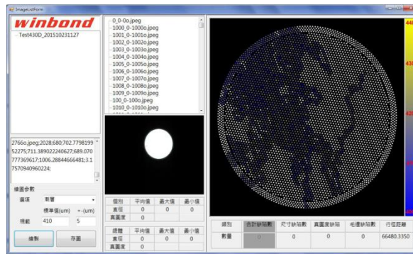
Shower Head AOI 檢測設備
